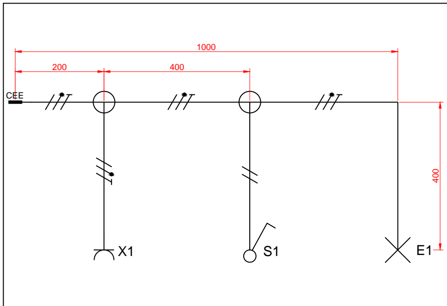
Installatieschema
